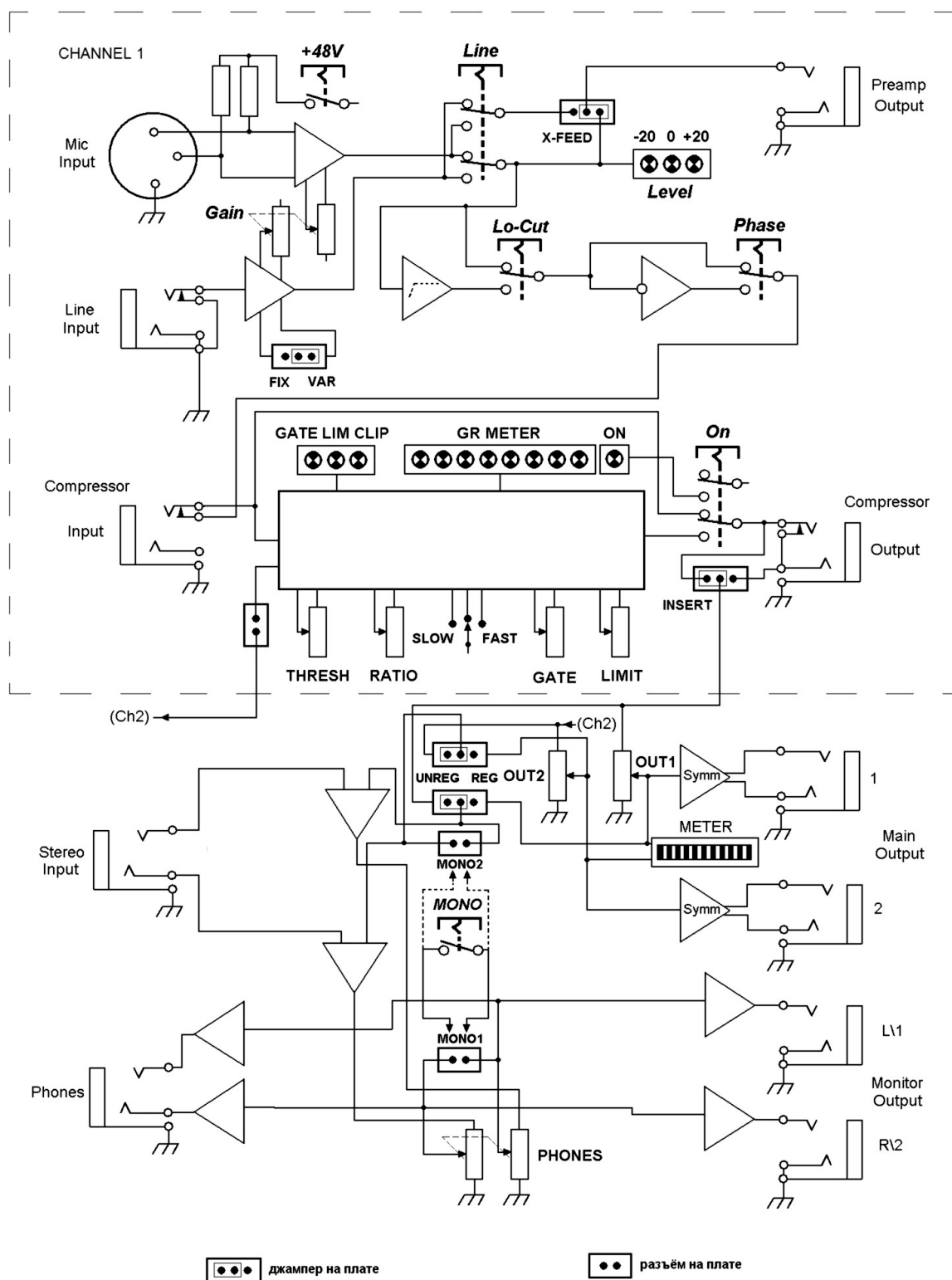
Упрощенная структурная блок-схема Stereo Channel.
